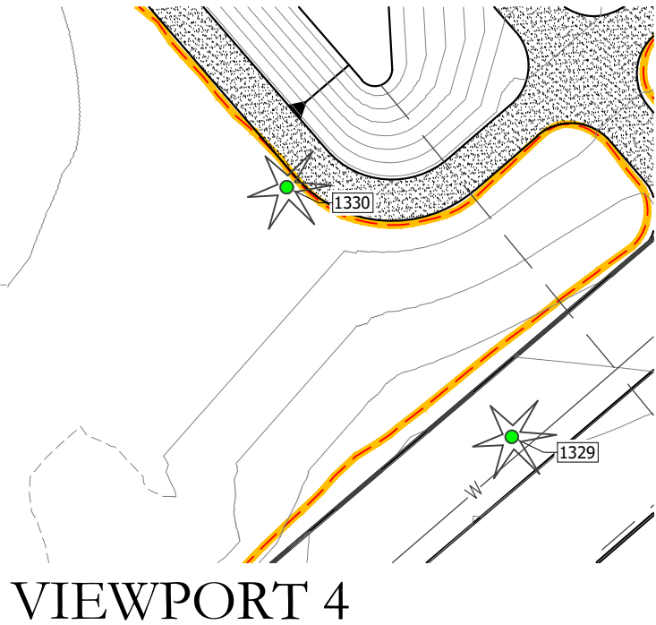
VIEWPORT 4 SCALE: 1"=50'
